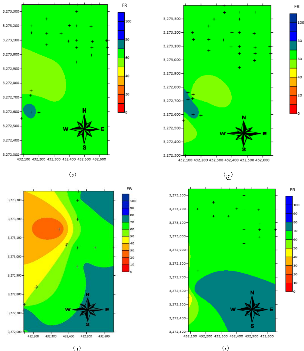
شکل 7 شبیه‌سازی متغیر جریان آب بازگشت حفاری به روش گوسی در تراز ارتفاعی 2729 (الف)، 2629 (ب)، 2579 (ج)، 2529 (د)، 2479 (ه) و 2429 (و) متر از سطح دریا
