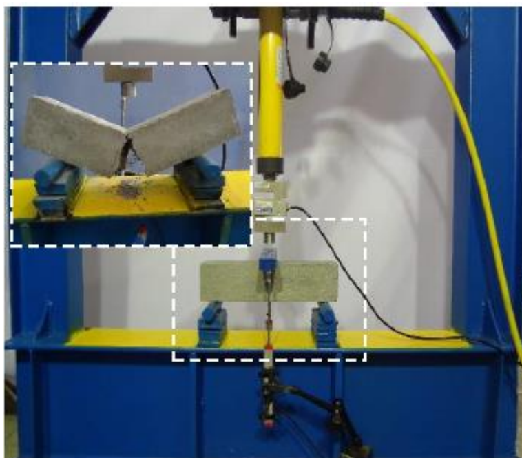
شکل ۷ انجام آزمایش خمش سه‌نقطه‌ای بر روی تیرها
