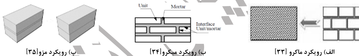
شکل ۹. رویکرد مدل‌سازی میان‌قاب مصالح بنایی
