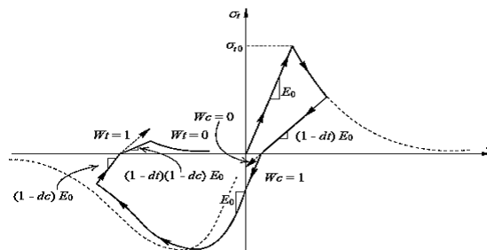
شکل ۱۰. رفتار بتن در بارگذاری تک محوره [۴۱]
