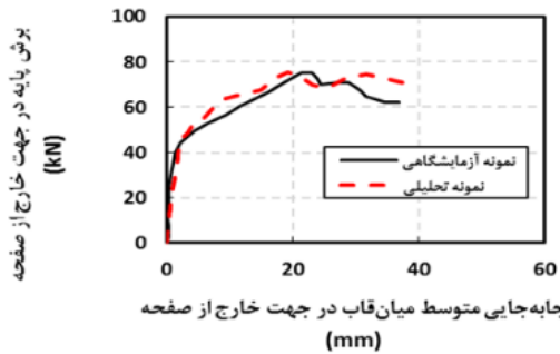
شکل ۱۳. مقایسه نمونه شاهد آزمایشگاهی با نمونه تحلیلی برای صحت سنجی بارگذاری خارج از صفحه
