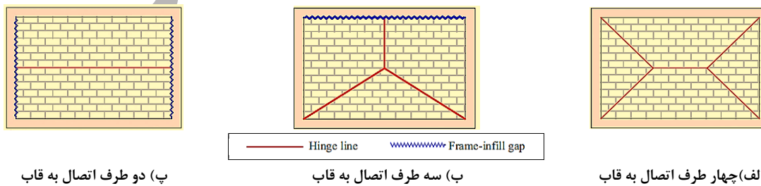
شکل ۵. عملکرد قوسی میان‌قاب مصالح بنایی در شرایط مرزی مختلف [۲۳]
