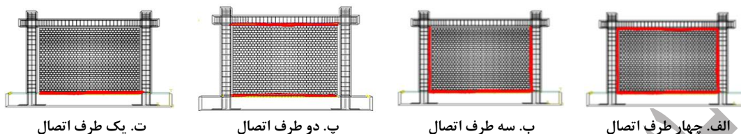
شکل ۸. شمای اتصال مختلف میان قاب به قاب بتن مسلح
