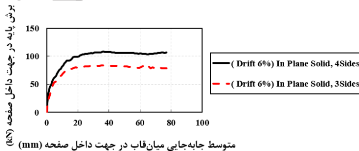
شکل ۱۹. مقایسه منحنی نیرو-جابه‌جایی در جهت داخل صفحه در قاب سه و چهار طرف اتصال
