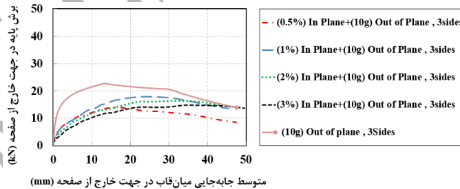
شکل ۱۷. تأثیر آسیب دیدگی داخل صفحه با جابه جایی نسبی مختلف بر مقاومت خارج از صفحه میان قاب با سه طرف اتصال
