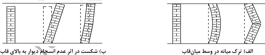
شکل ۴. حالت‌های مختلف شکست میان‌قاب در خارج از صفحه [۲۳]
