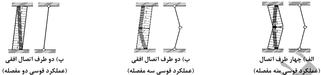
شکل ۳. عملکرد قوسی تحت شرایط مرزی مختلف [۳۰]
