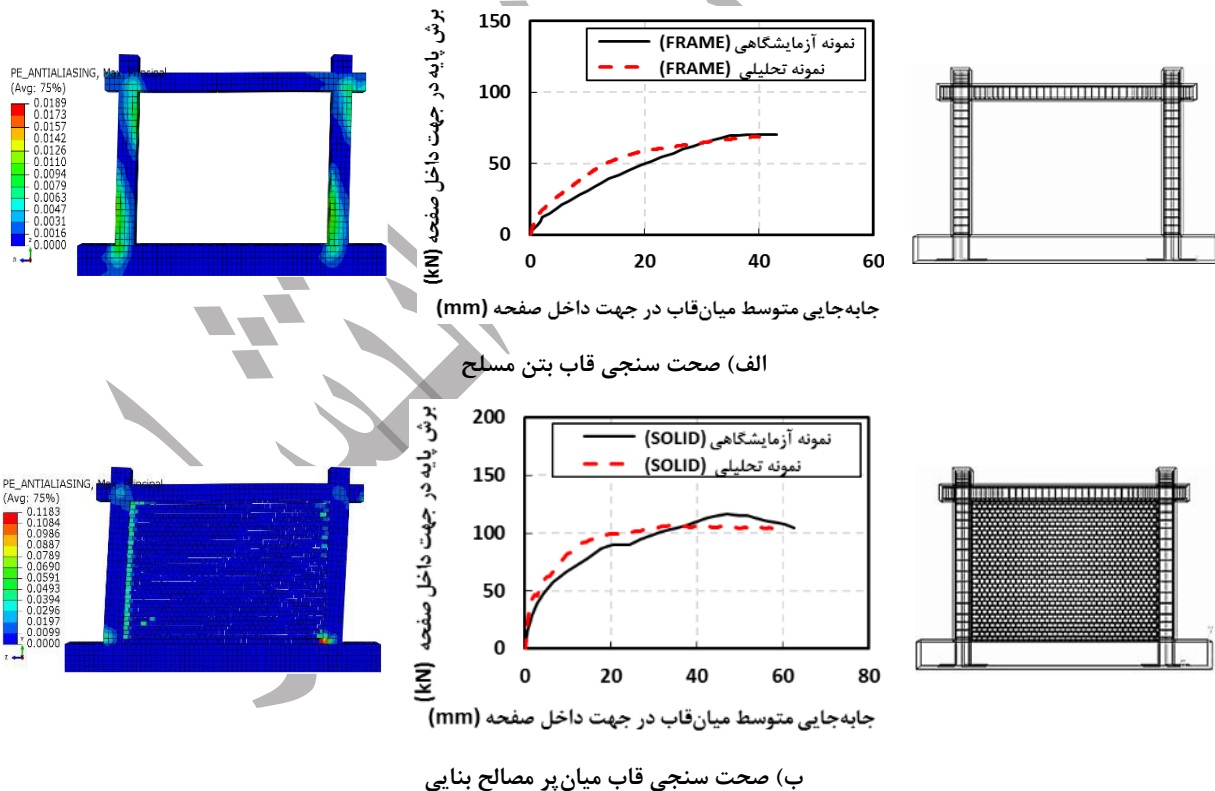
شکل ۱۲. مقایسه نمونه شاهد آزمایشگاهی با نمونه تحلیلی برای صحت سنجی بارگذاری داخل صفحه
