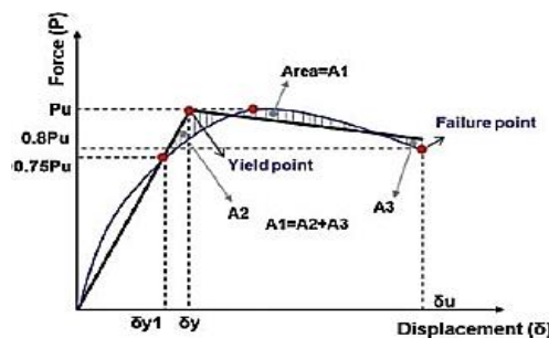
شکل ۱۱. دوخطی سازی نمودار نیرو-جابجایی [۴۴]
