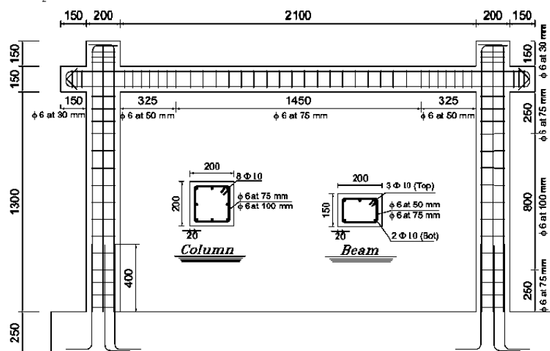
شکل ۶. ابعاد و جزئیات اجرایی قاب بتن مسلح (اندازه بر حسب میلیمتر) [۳۱]
