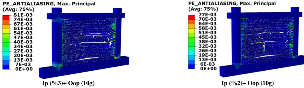
شکل ۱۶. تغییر شکل های پلاستیک و آسیب های نمونه قاب میان پر در چهار طرف اتصال
