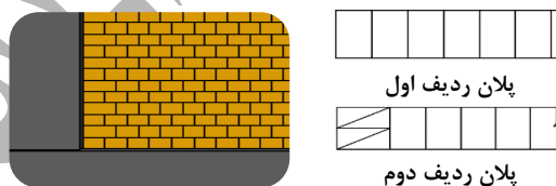
شکل ۷. الگوی آجر چینی قاب با میان قاب مصالح بنایی
